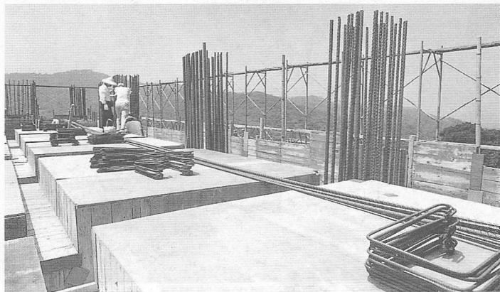
△中堂五樓頂層之鐵筋組合概況。
