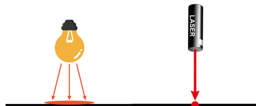
▲ 圖 2a（左）：普通光源匯聚點示意圖。 圖 2b（右）：雷射光源匯聚點示意圖。
